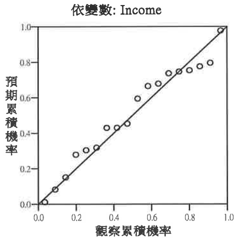
迴歸 標準化殘差的常態 P-P 圖
