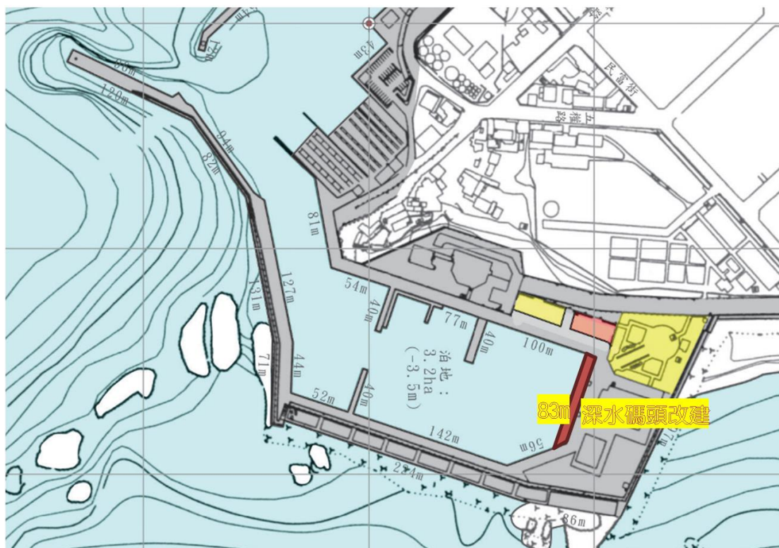
圖5-6-3 新港漁港深水碼頭工程位置圖
