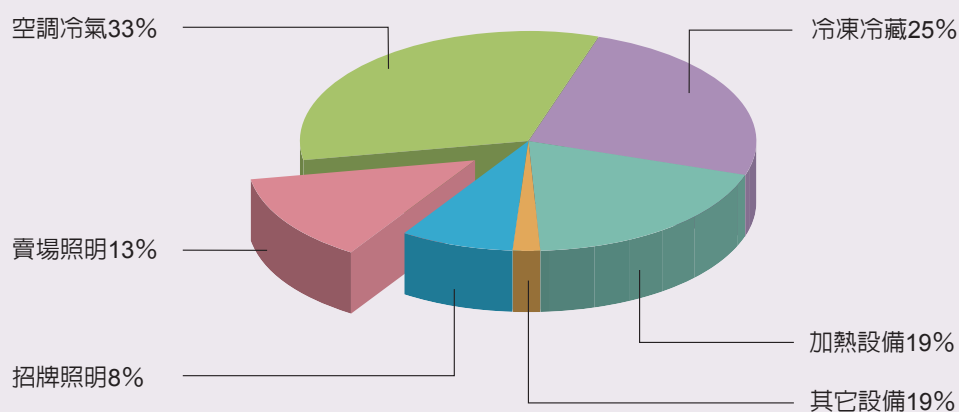
圖3 便利商店各類設備用電量比例圖
