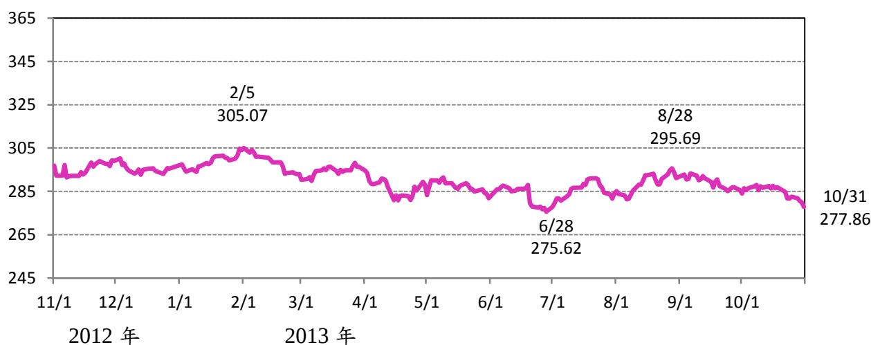
圖 4 CRB 走勢 (2012/11/1~2013/10/31)
