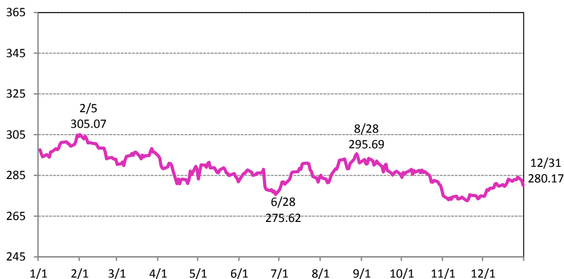
圖 4 CRB 走勢（2013/1/1~2013/12/31）
