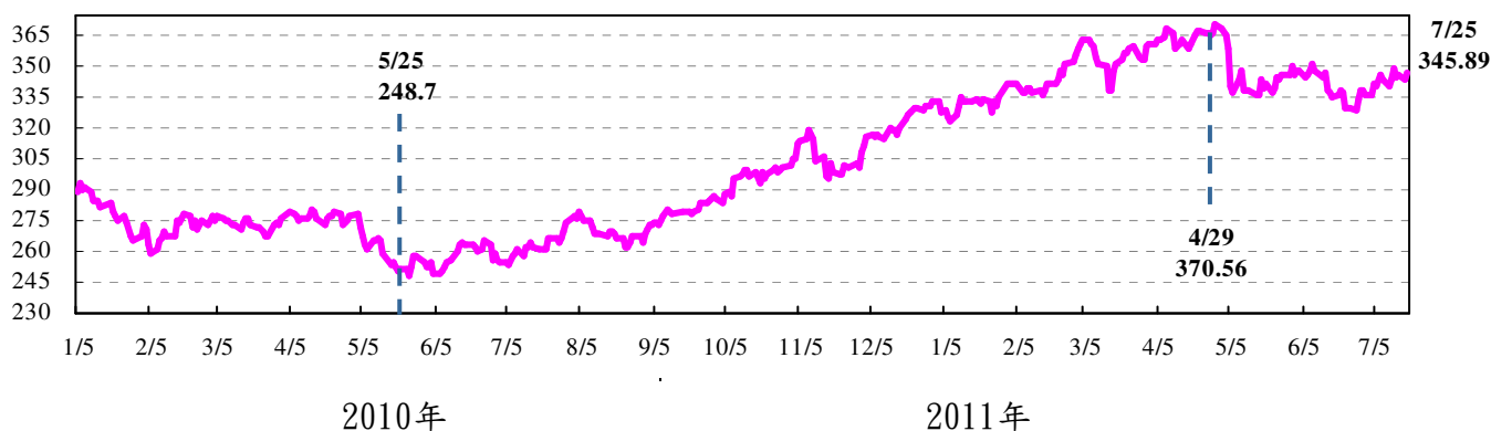
CRB 走勢 (2010/1/5~2011/7/25)
