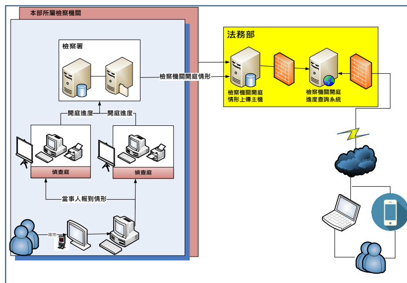
圖 1 系統整體架構圖
